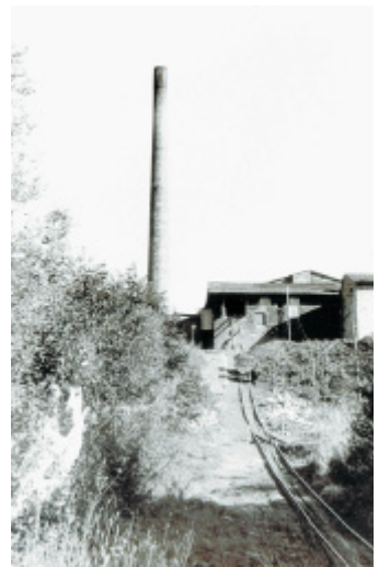
Lorenbahn: Auf Feldbahn-Gleisen wurde der Mergel zur Aufbereitung gefahren.
