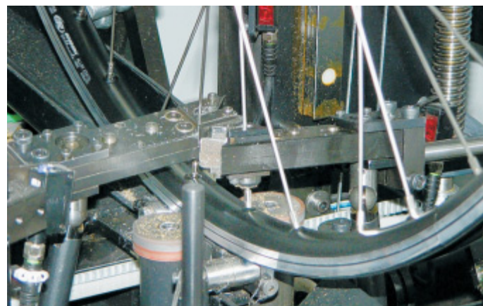
Zentrieren: Die Speichen eines Laufrads werden im Automaten gespannt und das Rad damit zentriert. Hier ist Handarbeit entbehrlich.
